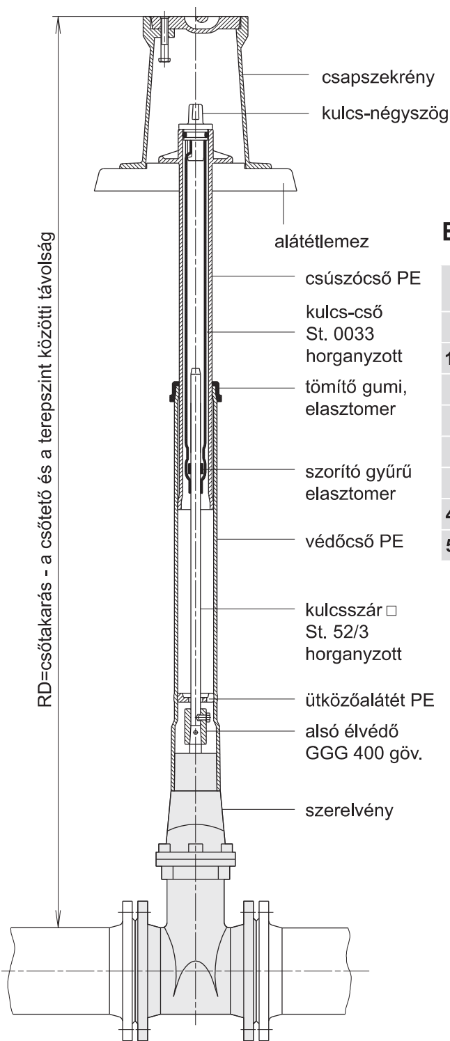
Ábra: teleszkópos beépítési készlet
